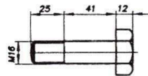
⑤ HEX BOLT MATL. M.S. QTY. = 4 Nos.
